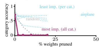
(d) causal pruning
