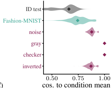
(d) far-OOD collapse
