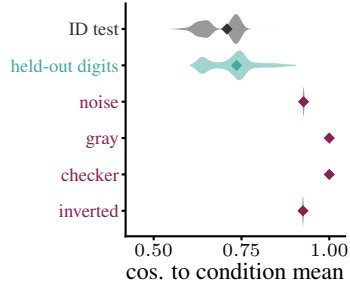
(d) far-OOD collapse
