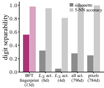
(d) digit separability
