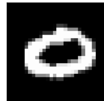
0 (even)
