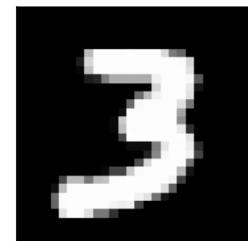
3 (odd)
