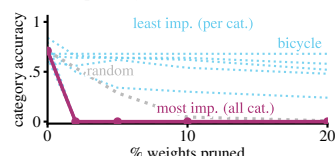
(d) causal pruning
