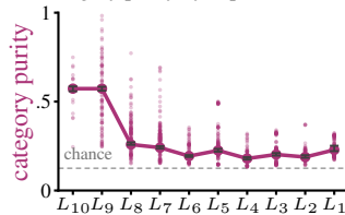
(d) category purity by depth
