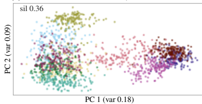
(h) ImageNet · classifier act., 512-d
