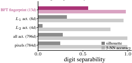
(d) digit separability
