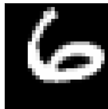
6 (even)
