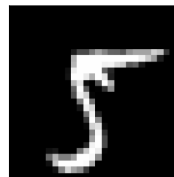
5 (odd)
