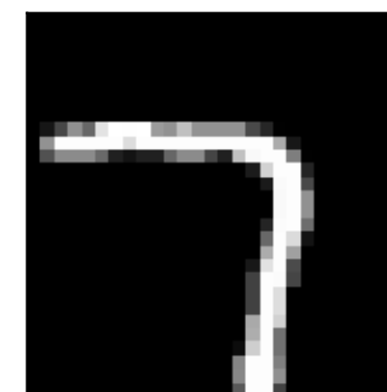
7 (odd)
