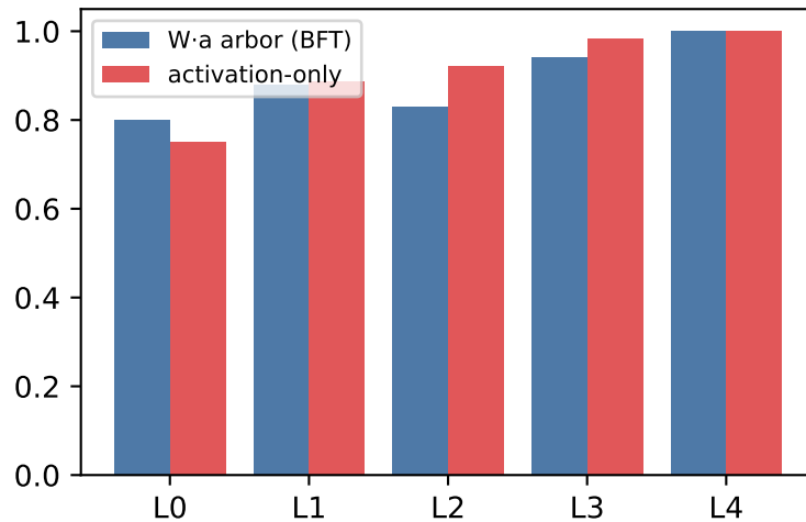
class selectivity (AUC)
