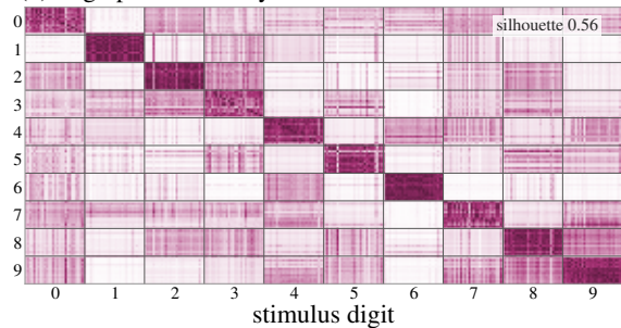
(d) fingerprint similarity
