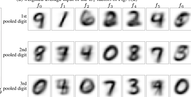
(d) weighted-average input of the L_1 factors of Fig. 3(d)
