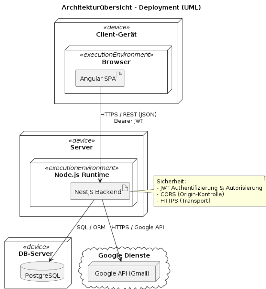
Abbildung 12: Architektordiagramm
