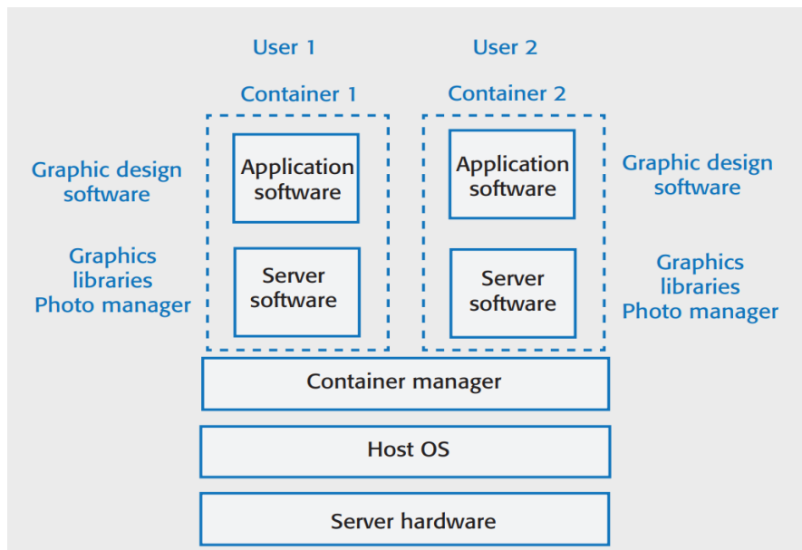
Abbildung 9: Aufbau Container - Cloud based Software Sommerville F. 8
