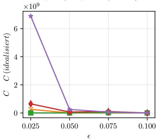
Barrier Option - Sprungadaptiert (Cutoff)
