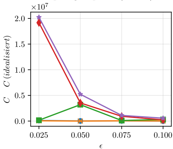
Asiatische Option - Sprungadaptiert (Cutoff)
