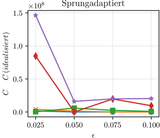
Barrier Option - Sprungadaptiert (Cutoff)
