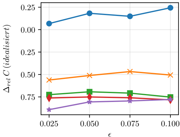
Barrier Option - Sprungadaptiert - Cutoff
