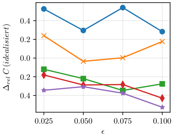
Asiatische Option - Festgitter - Cutoff
