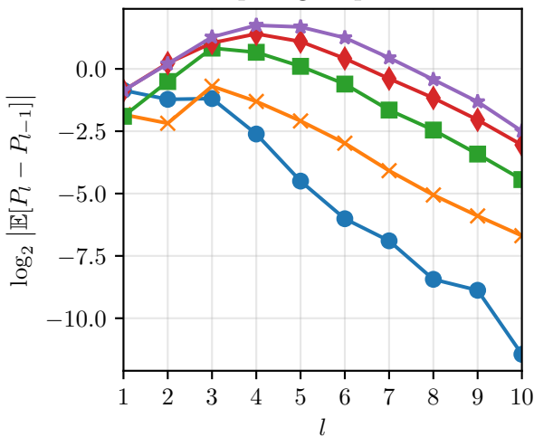
Barrier Option - Sprungadaptiert
