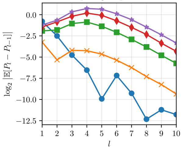
Asiatische Option - Sprungadaptiert
