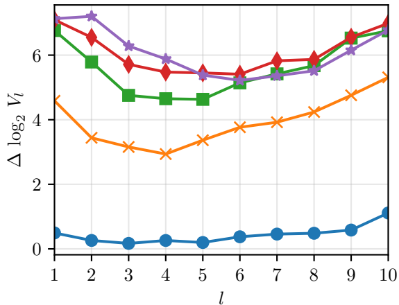
Asiatische Option - Sprungadaptiert - Cutoff
