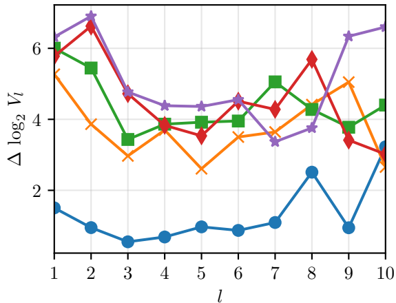
Barrier Option - Sprungadaptiert - Cutoff
