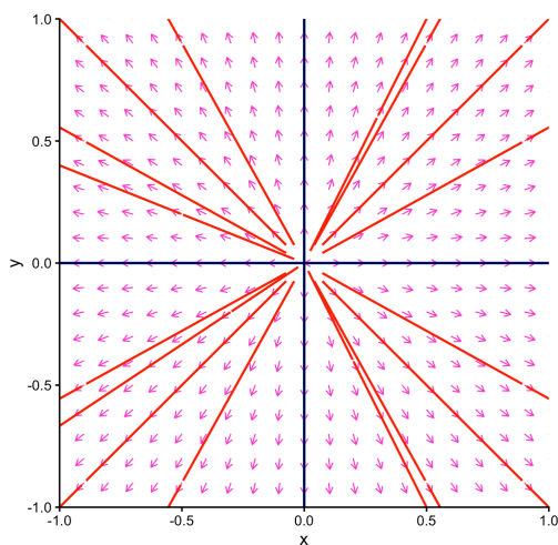
图 13: \mathbf{A} = \begin{pmatrix} 1 & 0 \\ 0 & 1 \end{pmatrix} , 此时 \mathbf{A} 有两个相同的正数特征值. 此时系统的稳定性取决于特征向量的符号. 因此 \mathbf{y}(t) = \mathbf{0} 不稳定.
