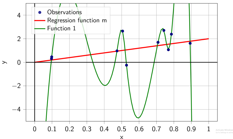
图 23: 利用 Lagrange 多项式和最小二乘分别对数据进行回归的比较. 在本图中观测到的数据点已用蓝色标出, 绿色曲线为 Lagrange 多项式的拟合结果; 红色直线为使用 y = \beta_0 + \beta_1 x + \varepsilon 得到的最小二乘拟合结果.
