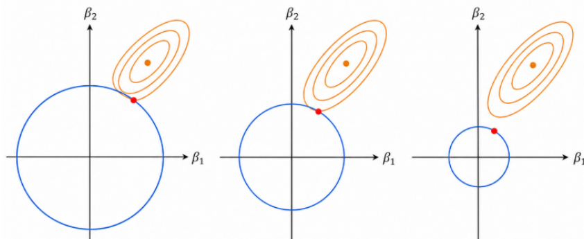
图 25: Ridge 回归的几何意义: 蓝色圆代表方程 \beta_1^2 + \beta_2^2 = \lambda^2 , 橙色的一簇簇椭圆既代表了函数 F(\beta) = \|\mathbf{y} - \mathbf{X}\beta\|^2 的等值线. 其中红色的点即为圆与等值线的切点. 红色切点越靠近椭圆的中心, 代表在此情况下数据的残差平方和越小.
