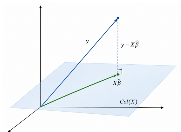
图 24: 最小二乘的几何关系: 满足 \|y - X\beta\| 最小的解即为 y 在设计矩阵 X 的列空间上的正交投影.
