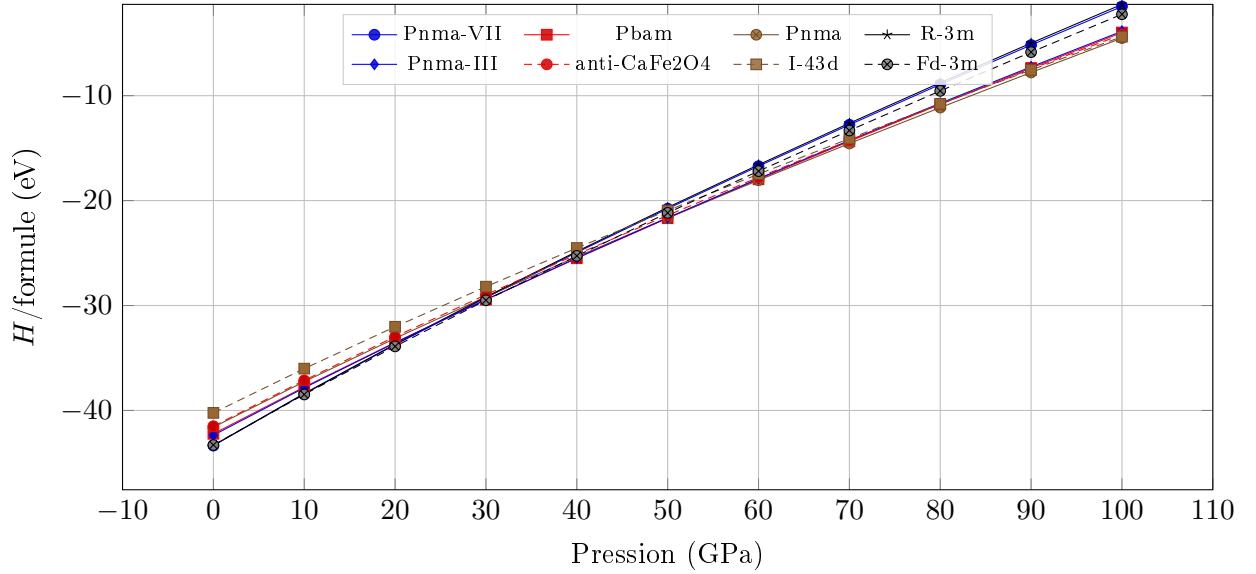
FIGURE 3 – Enthalpie H = E + PV par formule unitaire ( \text{Al}_4\text{C}_3 ) en fonction de la pression, pour les huit polymorphes. L’enveloppe inférieure (phase la plus stable à chaque pression) passe successivement par Pnma-VII (0–5 GPa), Fd-3m (5–32 GPa), Pbam (32–52 GPa) puis Pnma (52–100 GPa) – Fd-3m, initialement absent de ce diagramme, s’y révèle être la phase la plus stable sur près d’un tiers de la gamme de pression étudiée (voir section 3.6).
