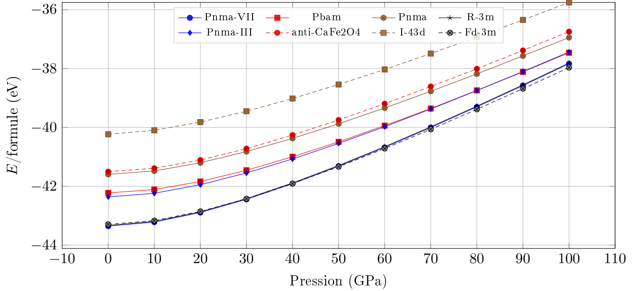
FIGURE 2 – Énergie totale (sans le terme PV ) par formule unitaire ( \text{Al}_4\text{C}_3 ) en fonction de la pression, pour les huit polymorphes. Contrairement à H(P) , l'ordre des courbes en E(P) reste globalement celui de P = 0 sur toute la gamme : c'est bien le terme PV (piloté par les écarts de volume, cf. figure 1) qui provoque les croisements observés sur le diagramme d'enthalpie.
