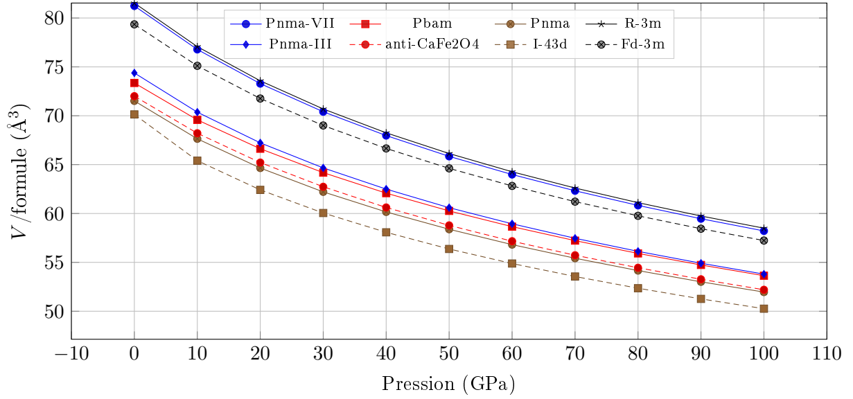
FIGURE 1 – Volume de la maille par formule unitaire ( \text{Al}_4\text{C}_3 ) en fonction de la pression, pour les huit polymorphes. Toutes les courbes décroissent de façon monotone et quasi parallèle : la compressibilité est similaire d’un polymorphe à l’autre, sans changement de pente marqué au voisinage des transitions de stabilité. Fd-3m ( 79.35 \text{ \AA}^3/\text{f.u.} à 0 GPa) se situe dans le haut du jeu, derrière R-3m et Pnma-VII, et suit la même loi de compression que les autres branches.
