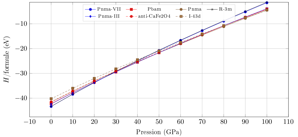
FIGURE 3 – Enthalpie H = E + PV par formule unitaire ( \text{Al}_4\text{C}_3 ) en fonction de la pression, pour les sept polymorphes. L'enveloppe inférieure (phase la plus stable à chaque pression) passe successivement par Pnma-VII, Pbam puis Pnma.
