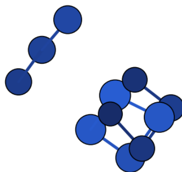
DFT (fragmentée, 3+8)
