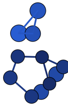
DFT (fragmentée, 3+8)
