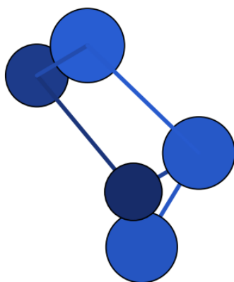
initiale (xTB, N_5^- intact)
