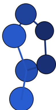
initiale (xTB, N_6^0 intact)
