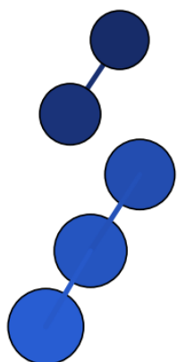
initiale (xTB, N 5 - intact)
