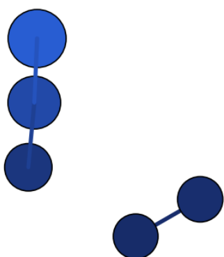
initiale (xTB, N 5 - intact)
