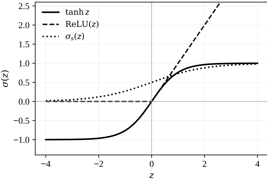
(a) Hàm kích hoạt
