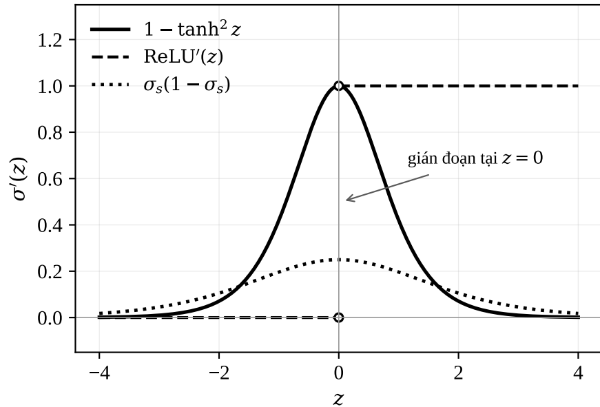
(b) Đạo hàm bậc nhất
