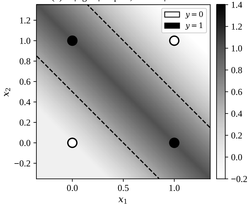
(b) Mạng một lớp ẩn, kích hoạt ReLU
