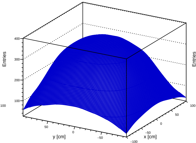
KDE
