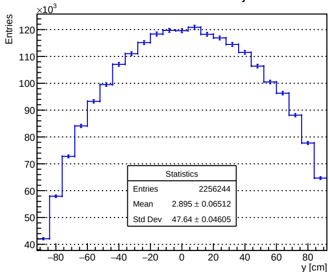
+100um x shift MM1 Y Projection
