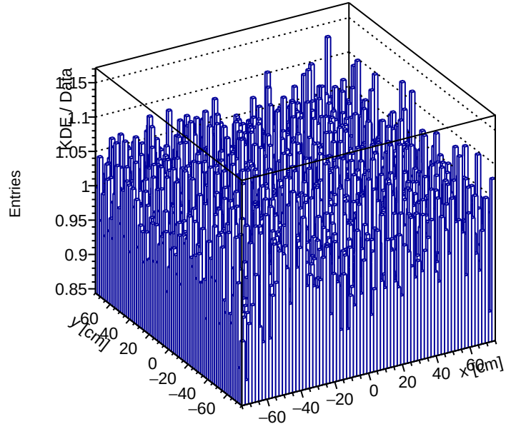
KDE / Data
