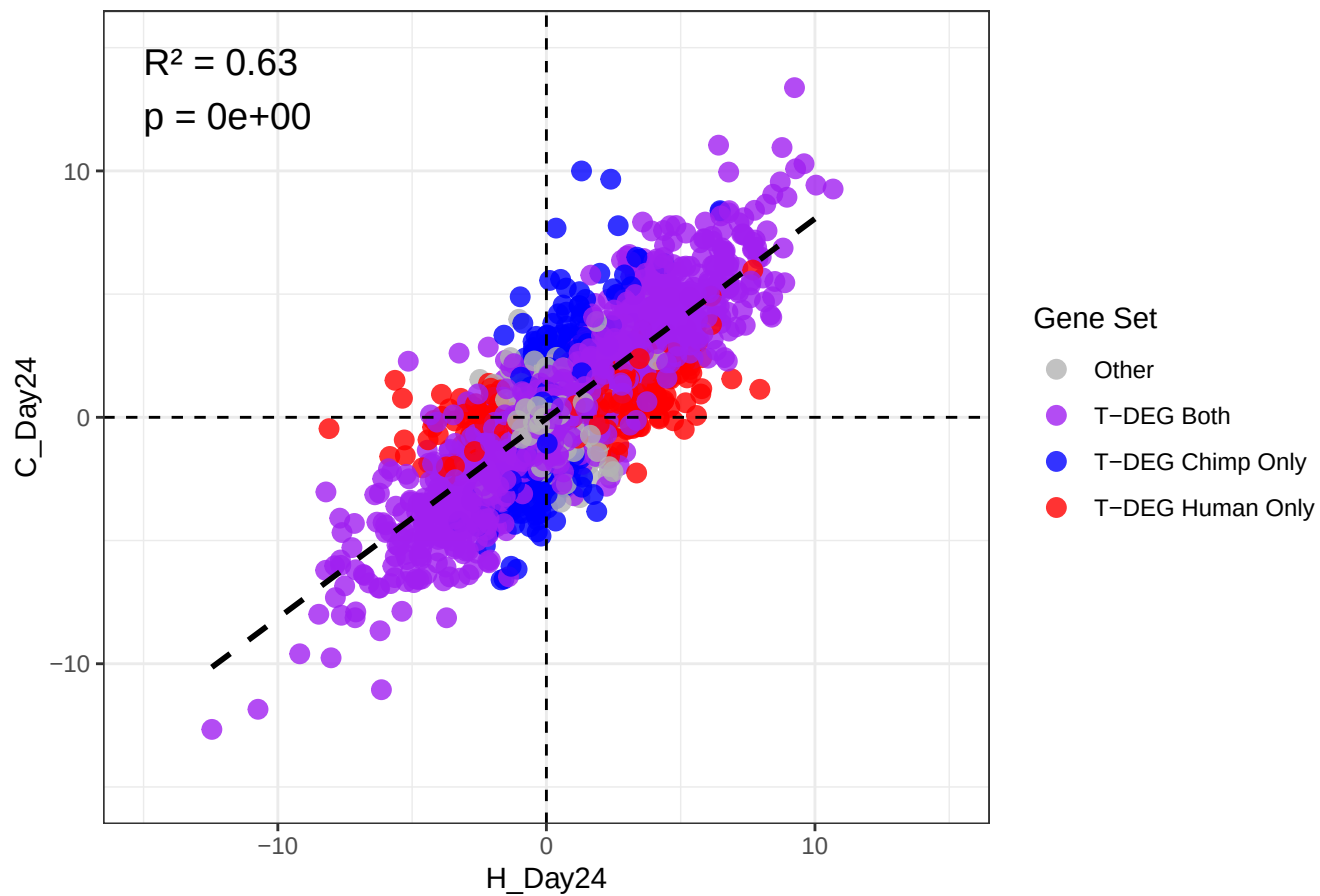
H_Day24 vs C_Day24 --All Expressed Genes
