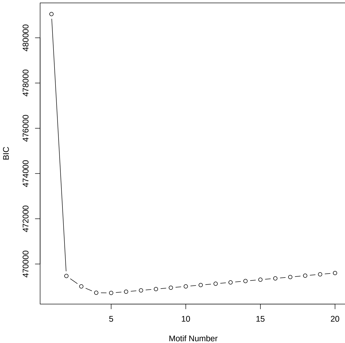
BIC
