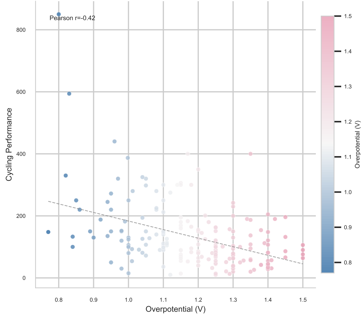
(d) Overpotential vs Cycling
