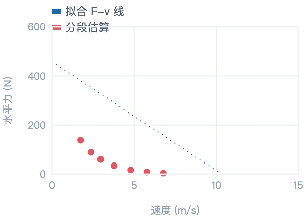
图 6b：水平力-速度剖面
