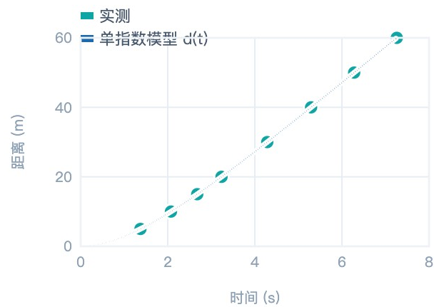
图 6a：距离-时间拟合
