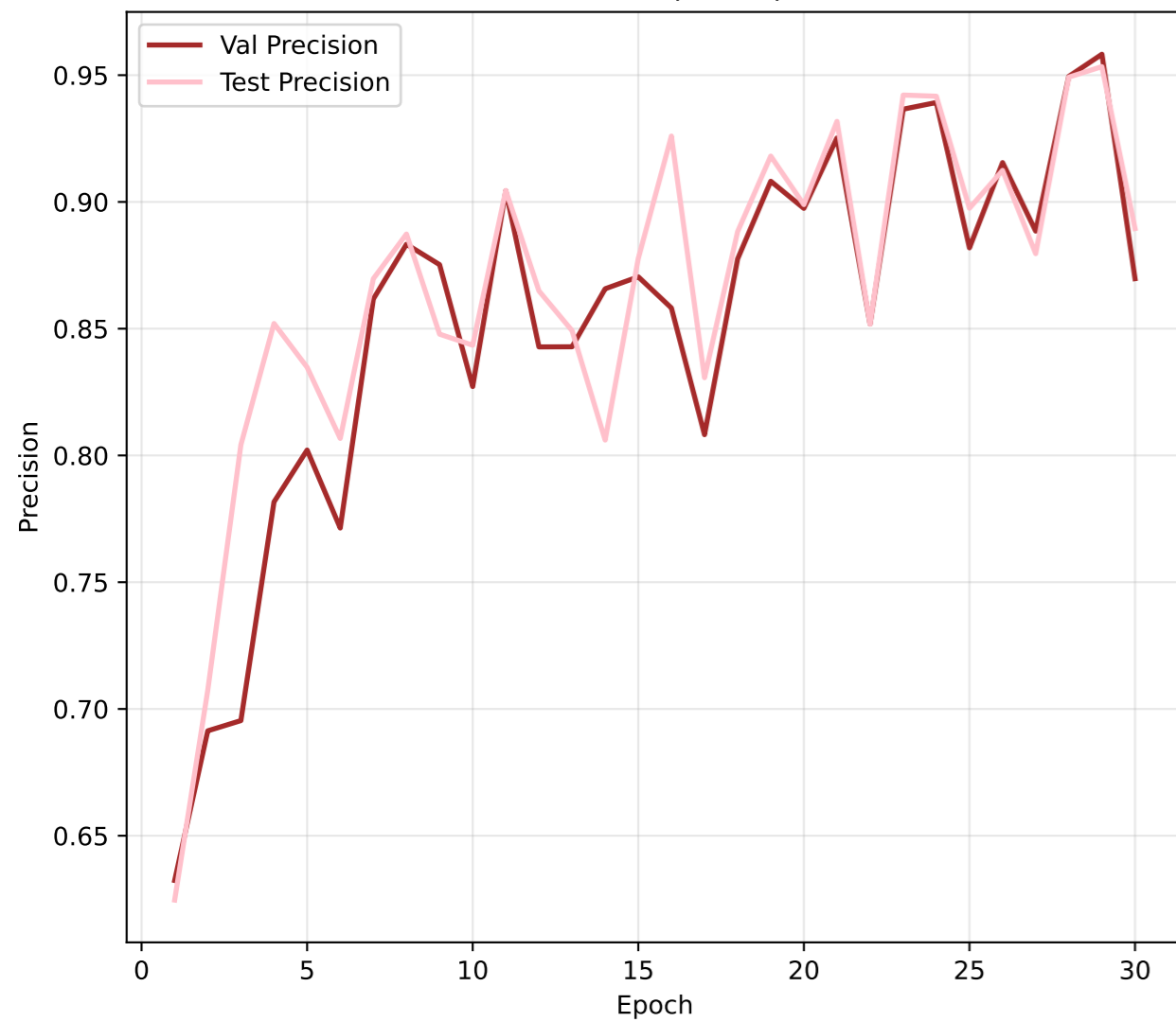
Precision (Macro)
