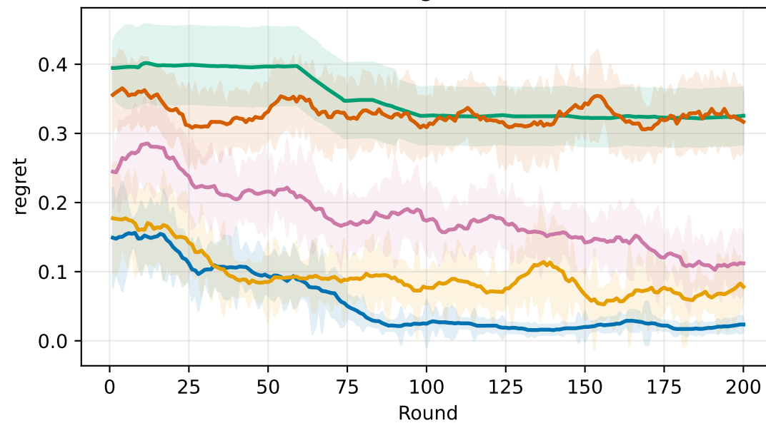
Regret
