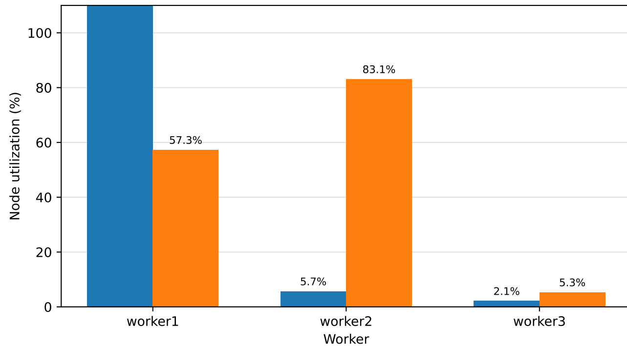
ResNet18EE
