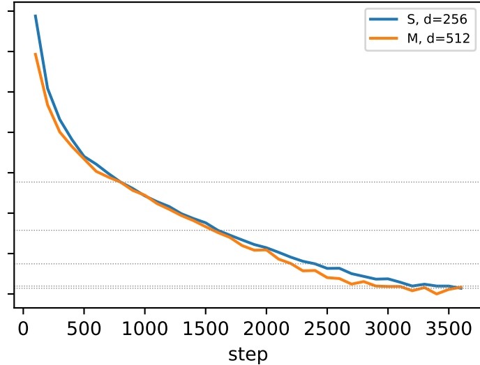
Study 2: lr 2.5e-4 (S), 5e-4 (M)
