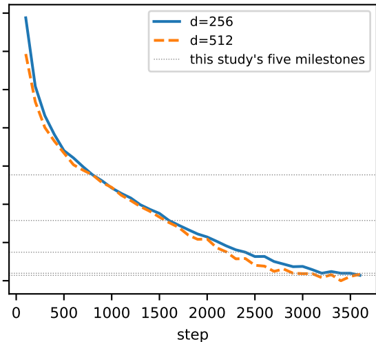
Study 2: rate 2.5 \times 10^{-4} (d=256), 5 \times 10^{-4} (d=512)
