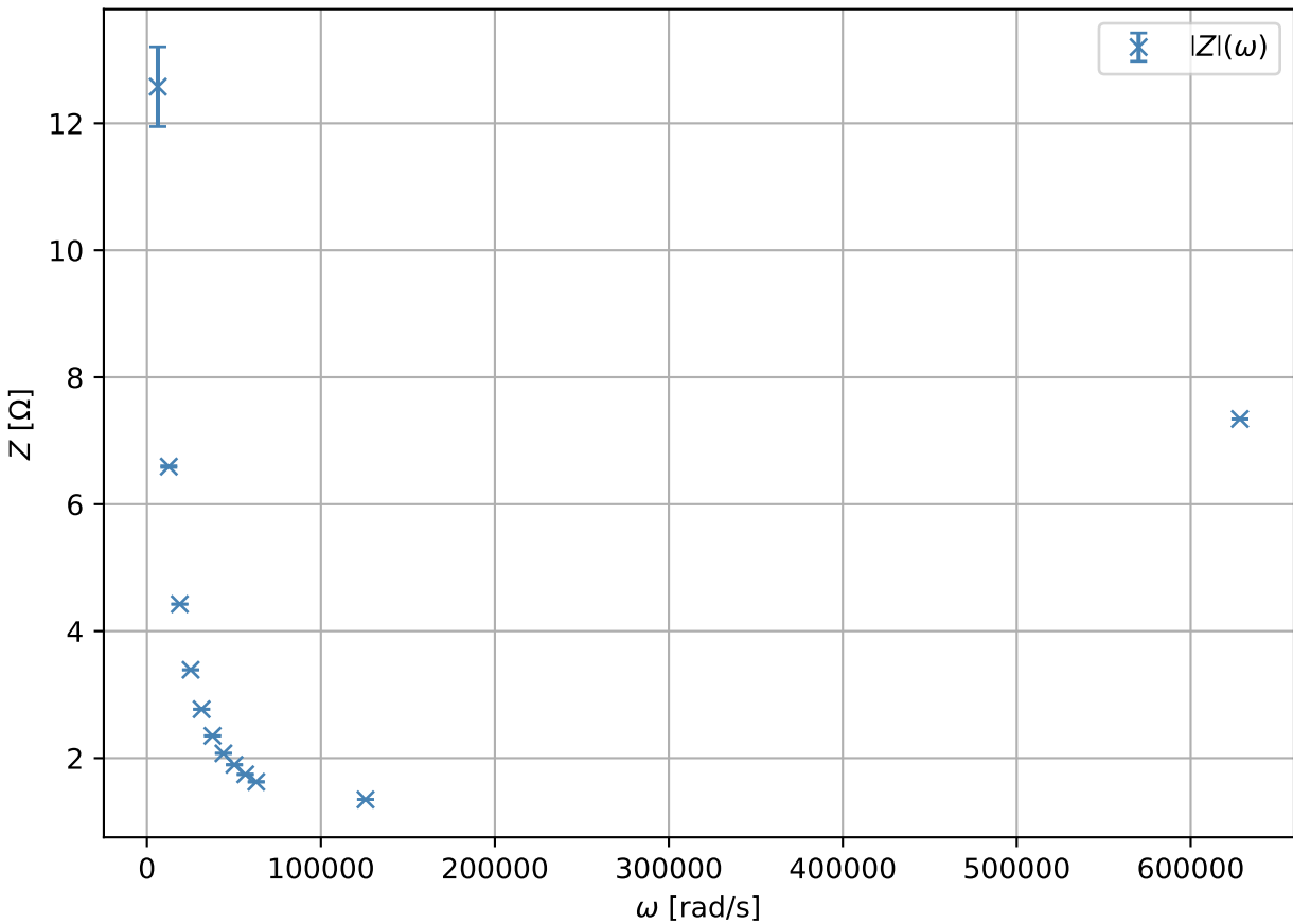
Impedanzbetrag |Z|(\omega)
