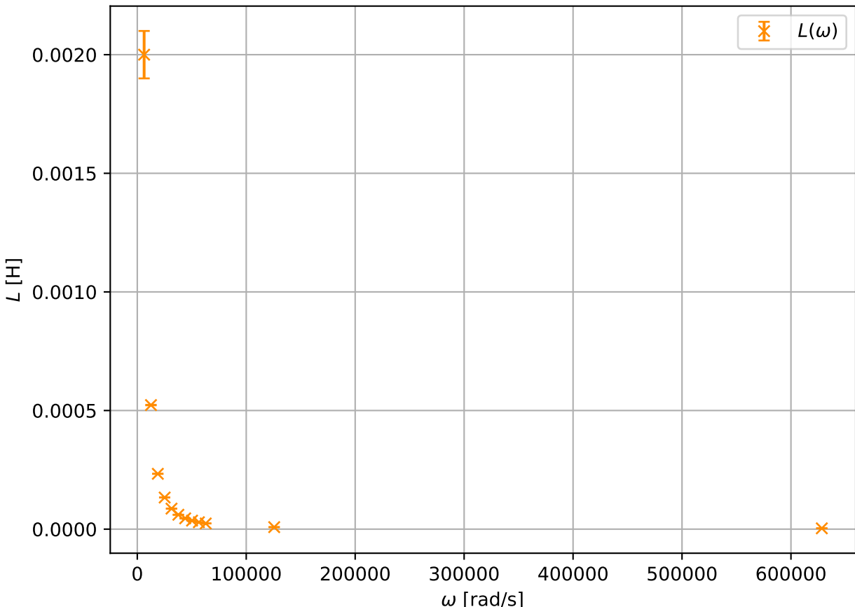
Induktivitätsbelag L(\omega)
