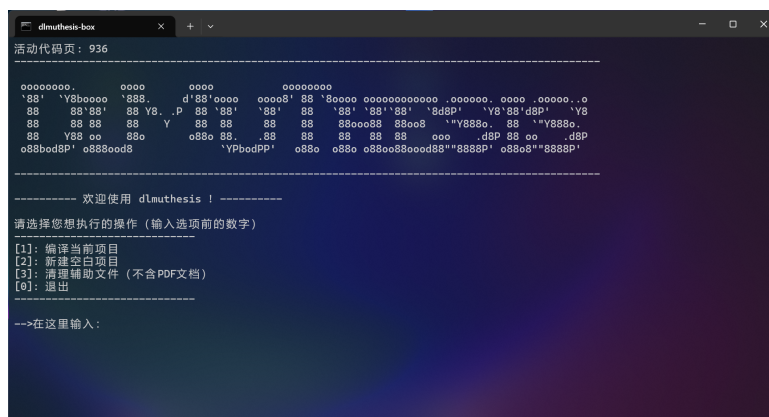
图 1: dlmuthesis-box 主界面
