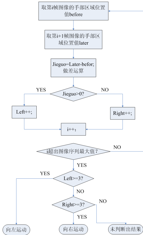
图 3.1 手势运动方向检测流程图
