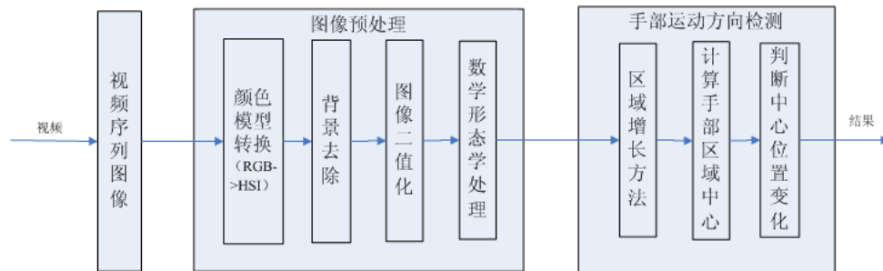
图 1.1 手部运动方向检测结构图
