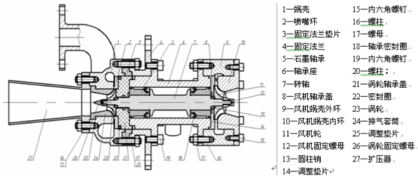
图 3.3 透平膨胀机的组成结构
