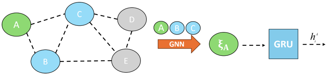
圖 3.5 GNN+GRU 架構
