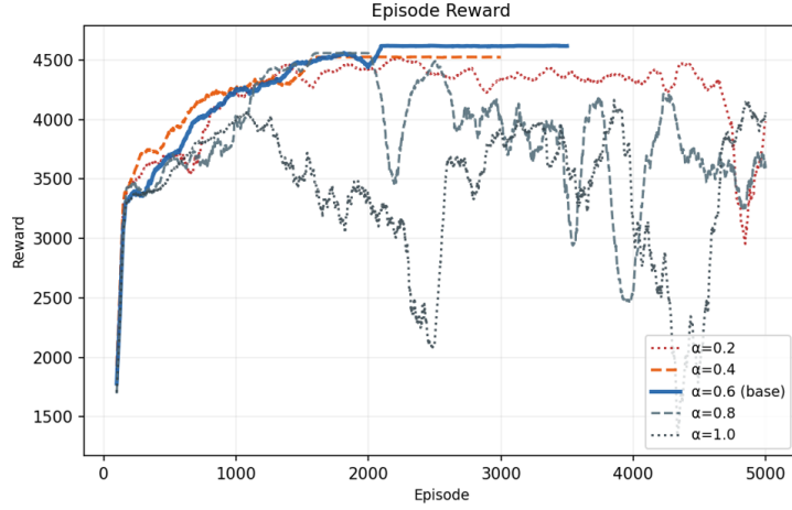
圖 5.10 各 a_{self} 訓練配置之 Reward 曲線
