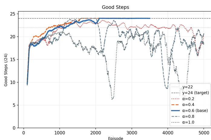
圖 5.9 各 a_{self} 訓練配置之 24 小時恢復曲線
