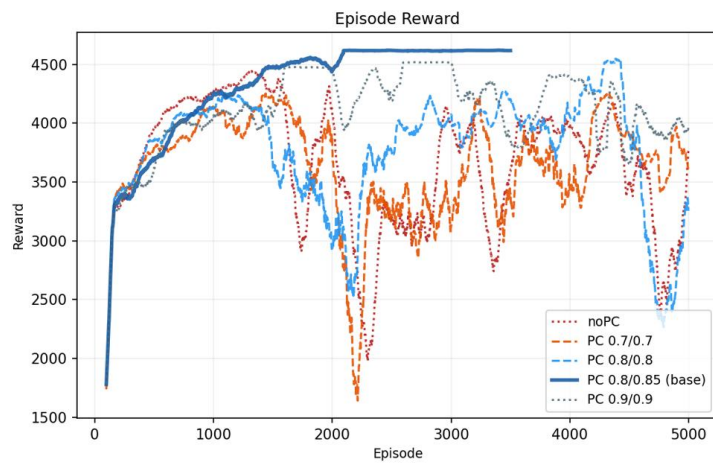
圖 5.8 各 PC 共識參數訓練之 Reward 曲線
