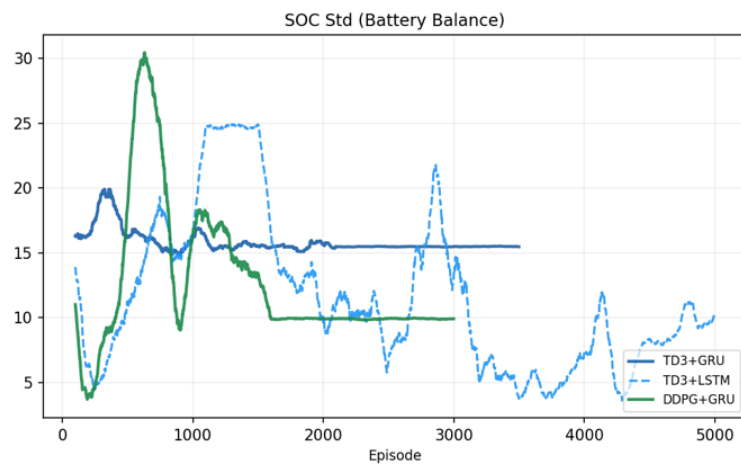
圖 5.3 固定初始 SOC 之 SOC std 曲線
