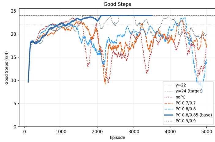
圖 5.7 各 PC 共識參數訓練之 24 小時恢復曲線
