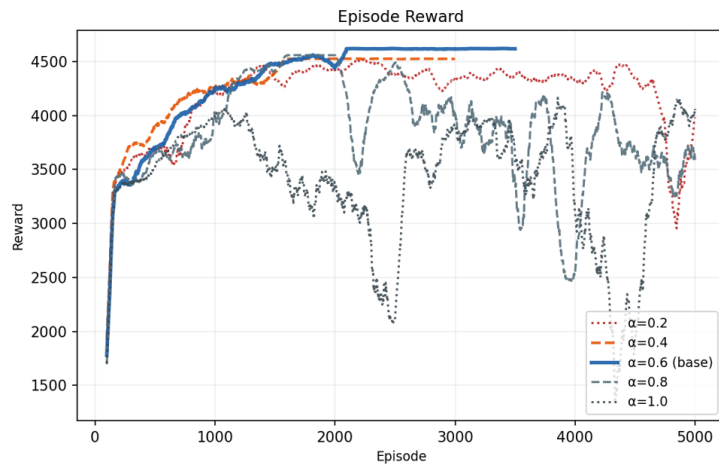
圖 5.11 各 a_{self} 訓練配置之 Reward 曲線
