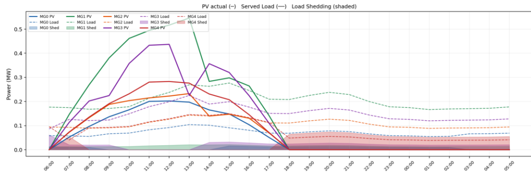
圖 5.13 PV 曲線、load 曲線、一般負載截斷量
