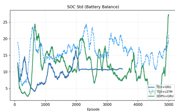
圖 5.6 隨機初始 SOC 之 SOC std 曲線
