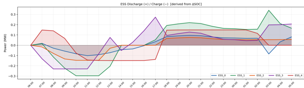
圖 5.15 SOC 充/放電曲線
