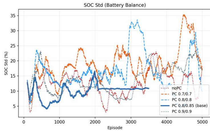
圖 5.9 各 PC 共識參數訓練之 SOC std 曲線
