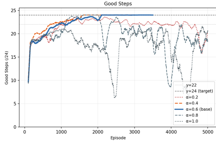
圖 5.10 各 a_{self} 訓練配置之 24 小時恢復曲線
