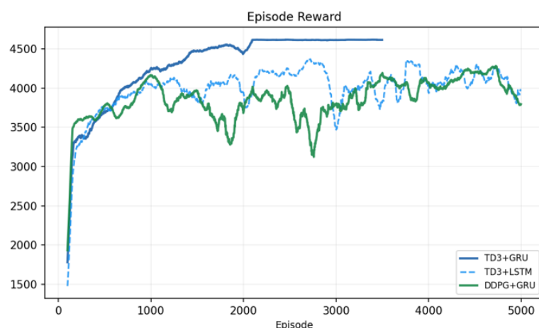
圖 5.5 隨機初始 SOC 之 Reward 曲線
