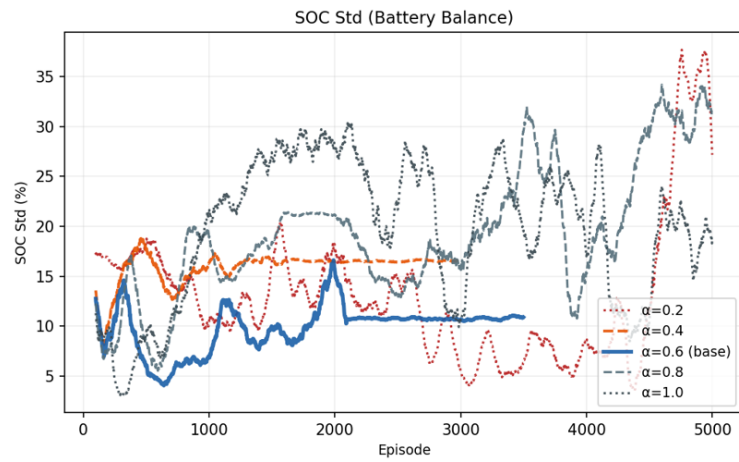
圖 5.12 各 a_{self} 訓練配置之 SOC std 曲線
