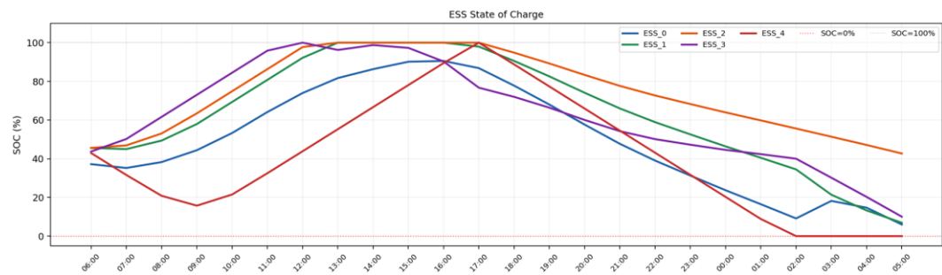
圖 5.14 SOC 電量曲線
