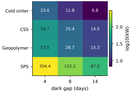
c Storage-equivalent power
