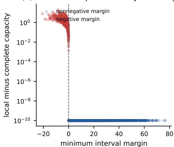
(d) Certificate separates every audited gap
