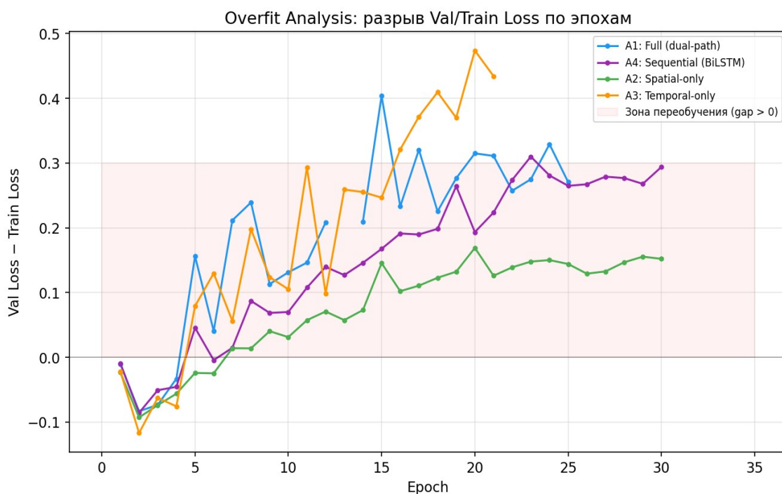
Рисунок 4.8 - Overfit analysis: разрыв Val/Train Loss по эпохам
