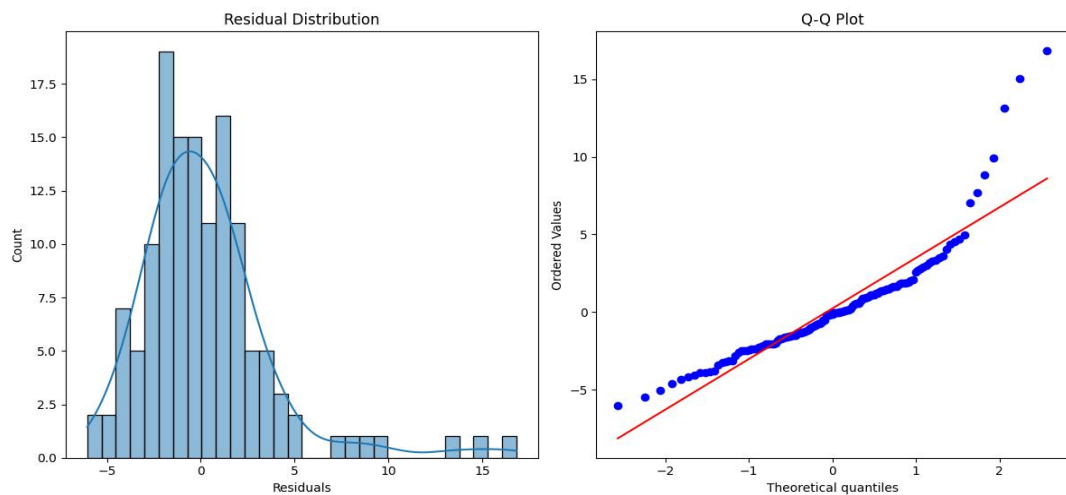
图10 二号线残差分布图（左）Q-Q Plot（右）
