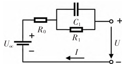
图 1 Thevenin 等效电路模型
