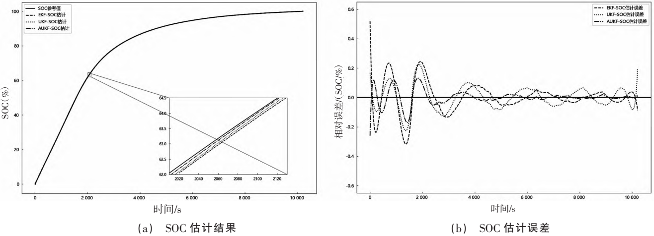
图 3 NASA 锂离子电池充电 SOC 估计
